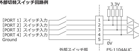
外部切替スイッチ回路例
