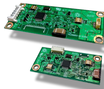
コントロールボード（USB） シングル入力用（上） シングル/デュアル入力用（下）
