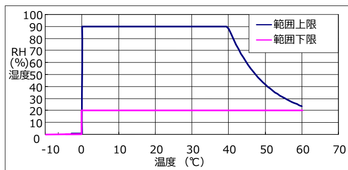
図-1 動作温湿度範囲
